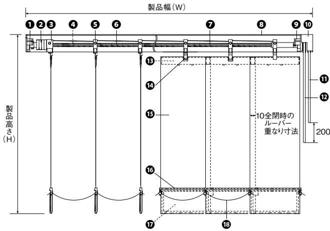
正面図
