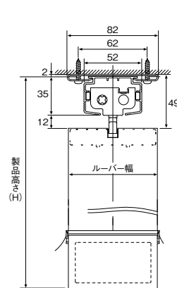
天井付け (天井付ブラケット使用)
