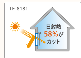
パーチカルブラインドを付けた場合 複層ガラス窓 + パーチカルブラインド \eta = 0.42 (TF-8181)
