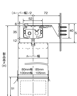
正面付け (正面付ブラケット使用)
