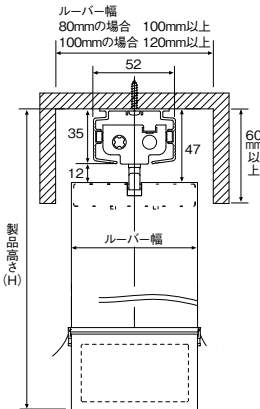
カーテンボックスの内側に取付ける場合
